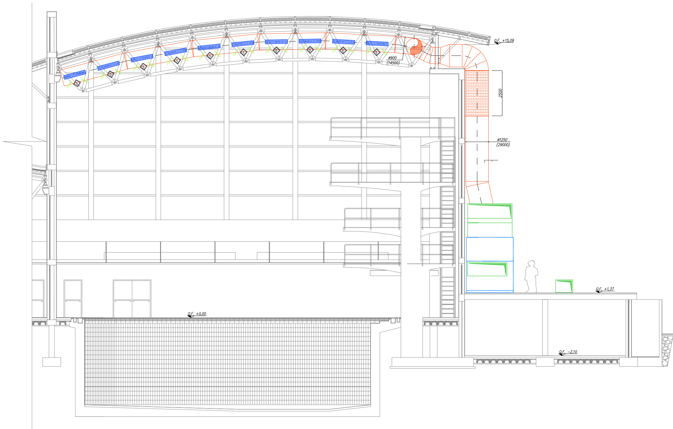
SEZIONE A-A
