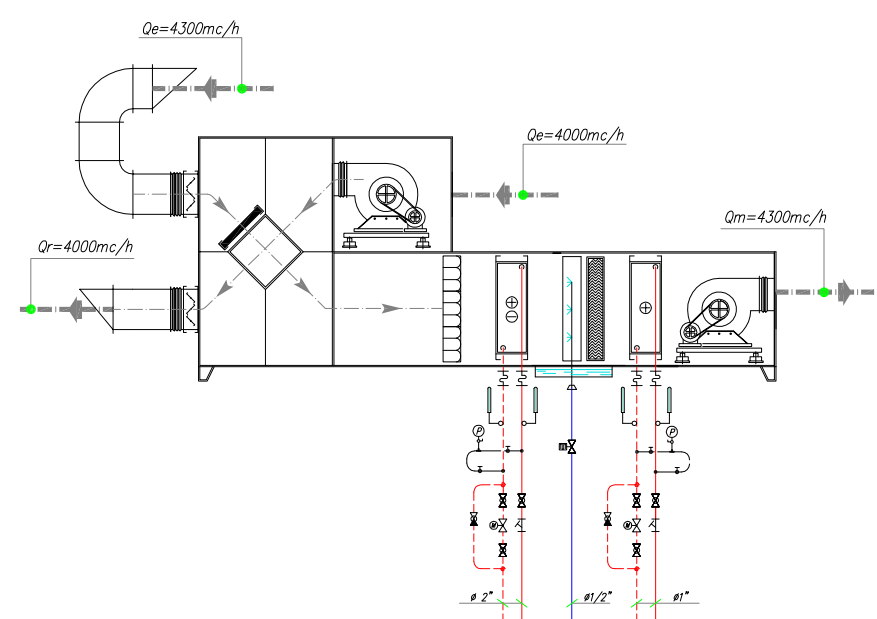
UTA PER IMPIANTO ARIA PRIMARIA CON RECUPERO STATICO
