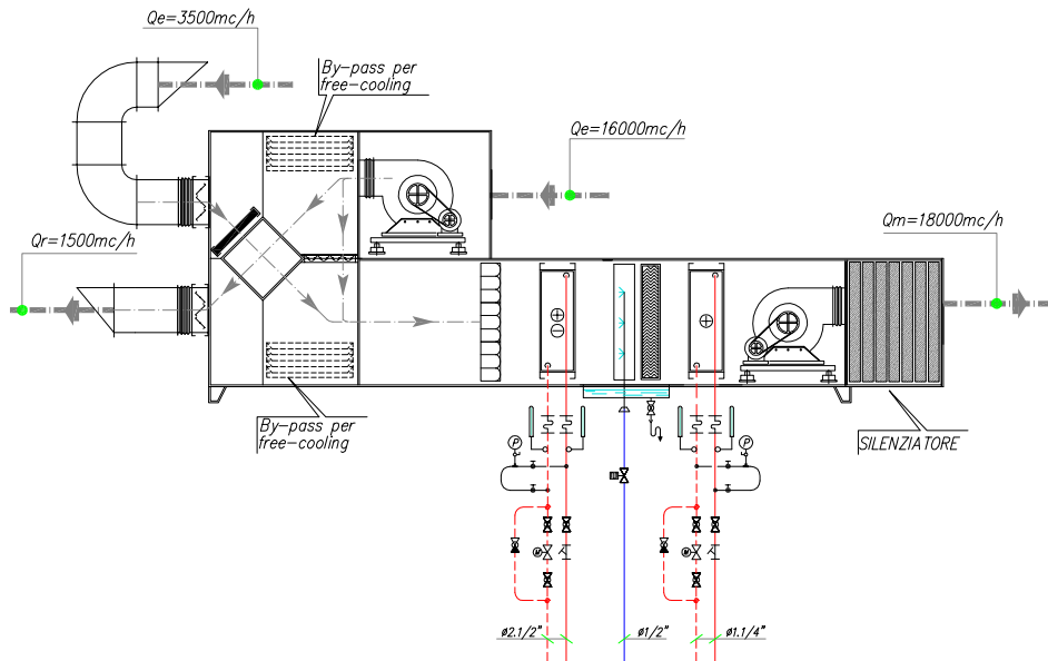
UTA PER IMPIANTO A TUTT'ARIA E FREE COOLING
