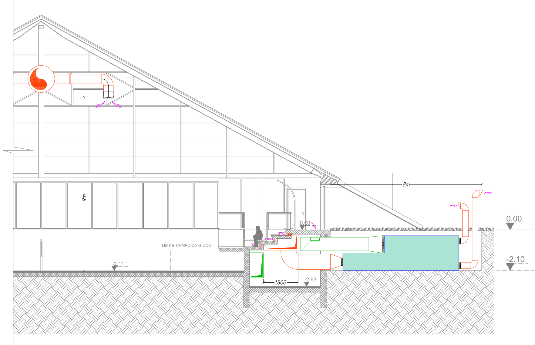
SEZIONE A-A
